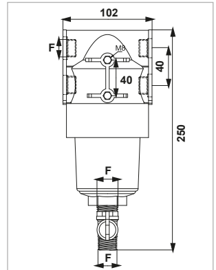
Kelebek Vana Ball Valve Válvula de bola 09003703
